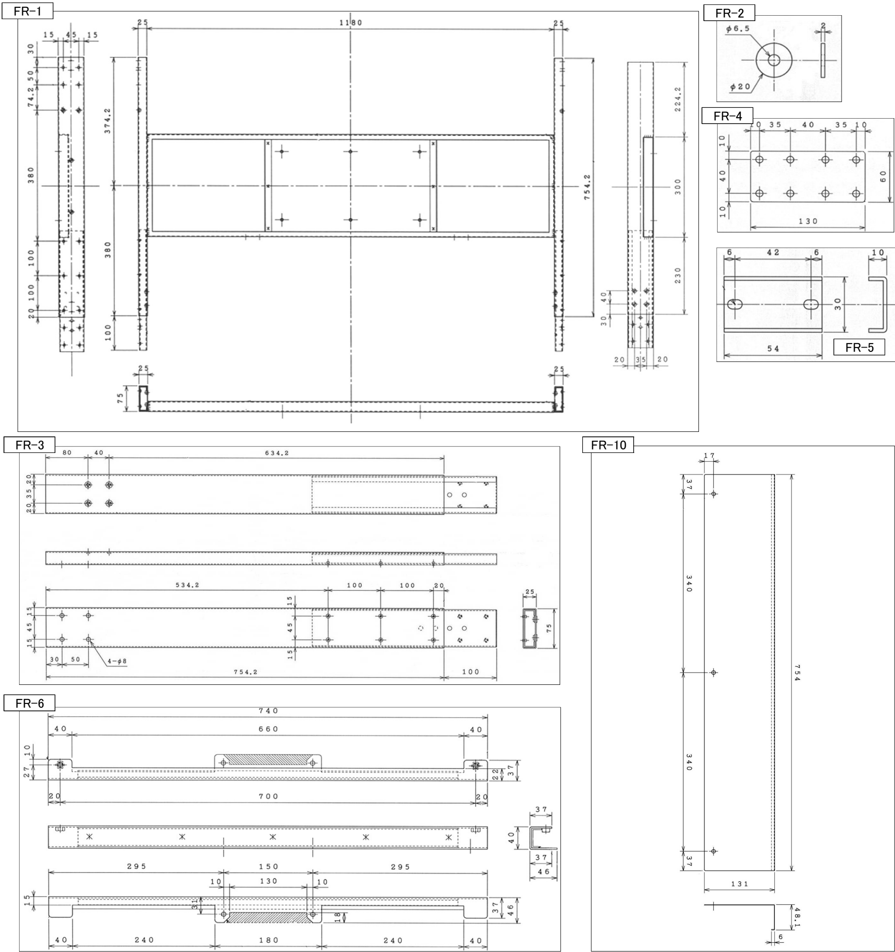
仕 様 図
