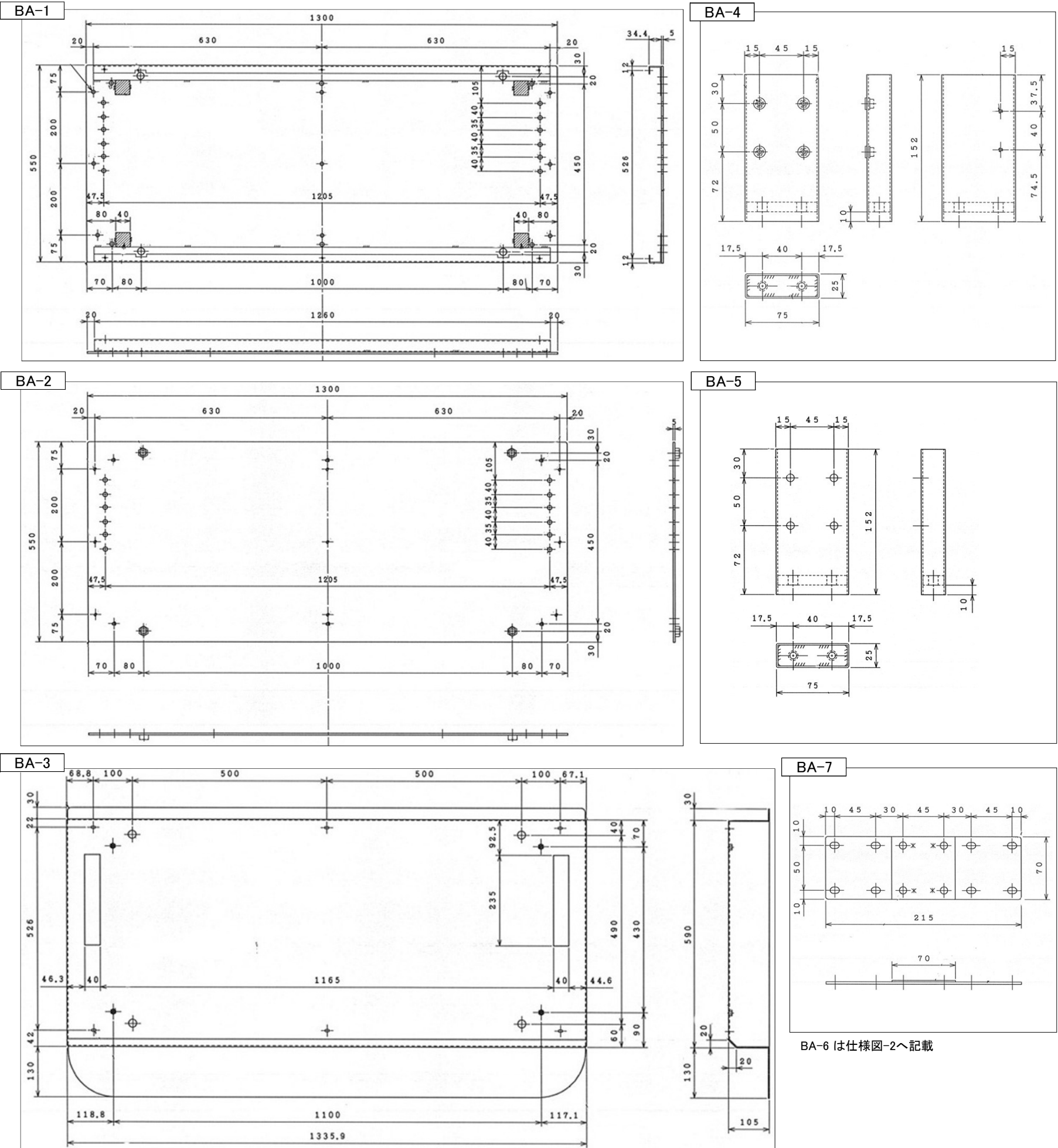
仕 様 図 - 1
