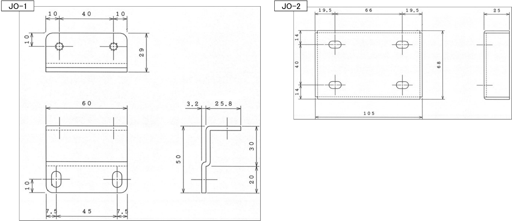
仕 様 図
