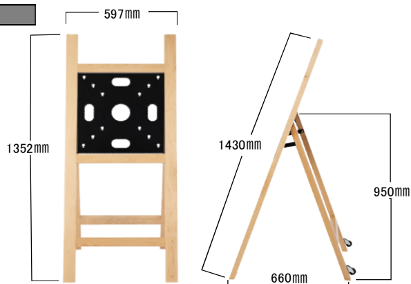
寸法図
